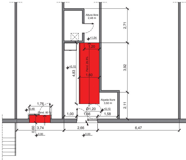
ZONA D'ACTUACIÓ INTERIOR - ESTAT FINAL (SENSE OCUPACIÓ A LA VIA PÚBLICA) NO VIABLE - PENDENT 29,8% EN RAMPA
