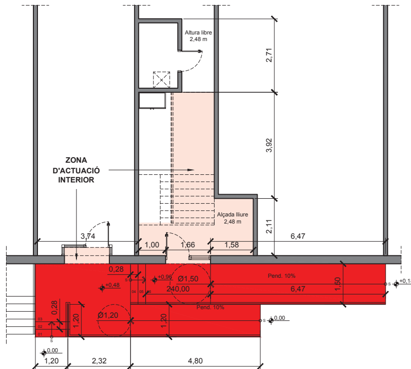
ZONA D'ACTUACIÓ EXTERIOR - ESTAT FINAL ESC. 1/100
