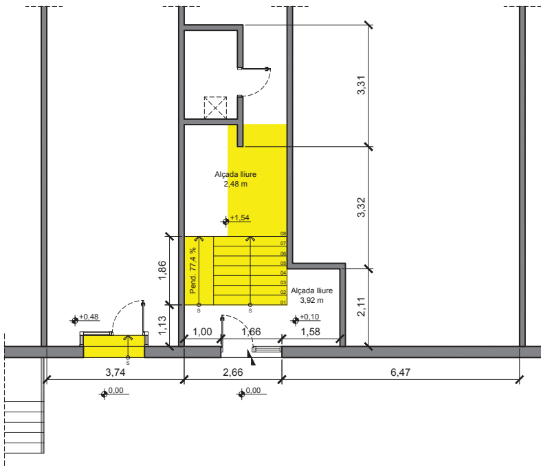
ZONA D'ACTUACIÓ INTERIOR - ESTAT ACTUAL (SENSE OCUPACIÓ A LA VIA PÚBLICA)
